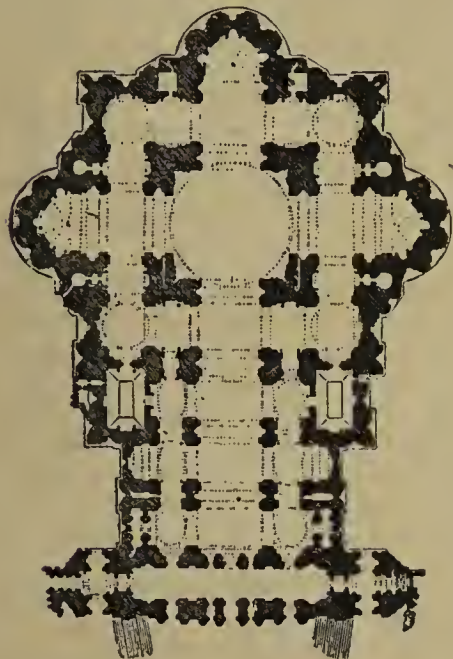
FIGURA 310—(Springer, o. c.), Planta actual de la basílica de San Pedro.
